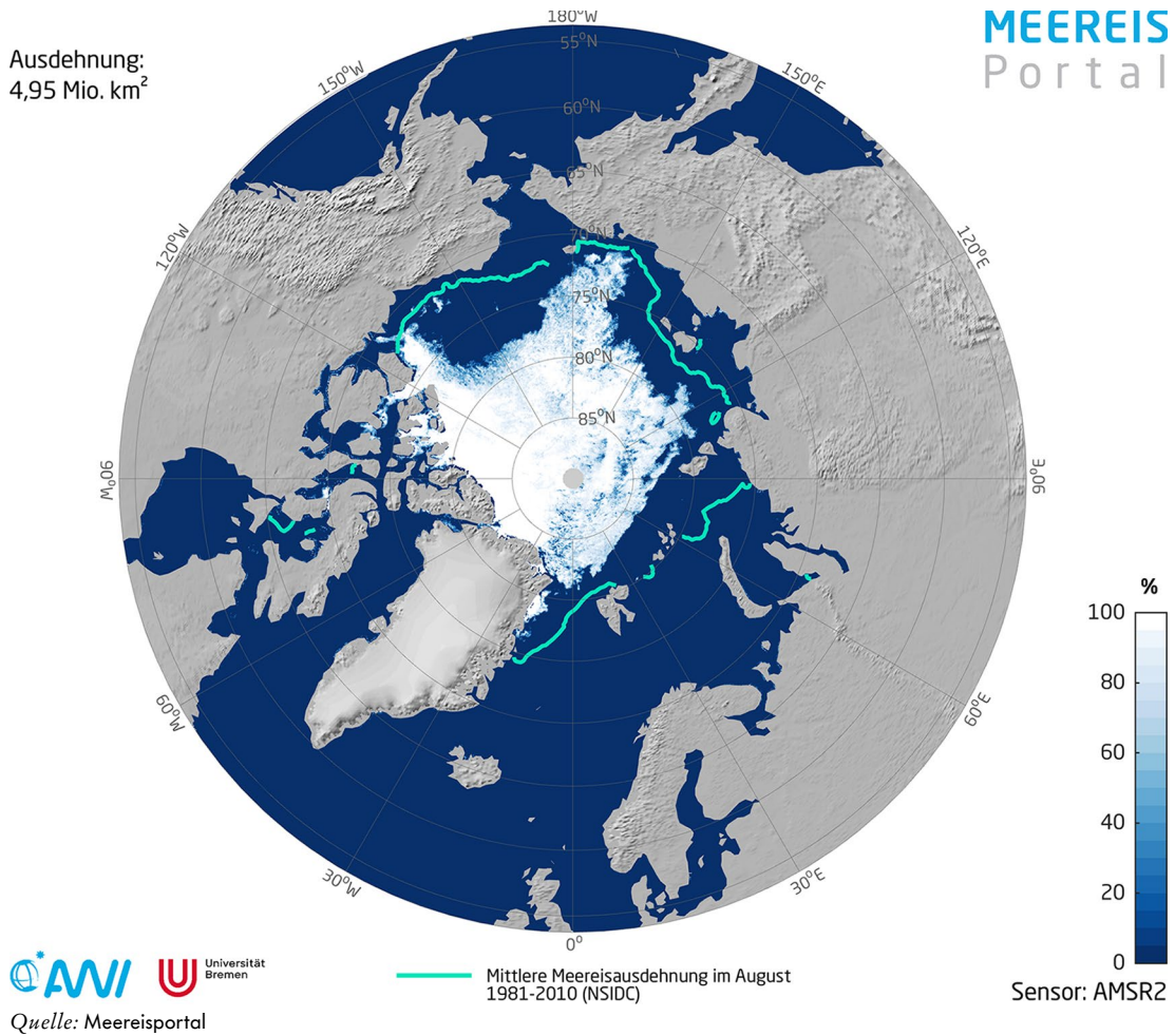
Abbildung 2: Meereiskonzentration in der Arktis am 31.8.2025
