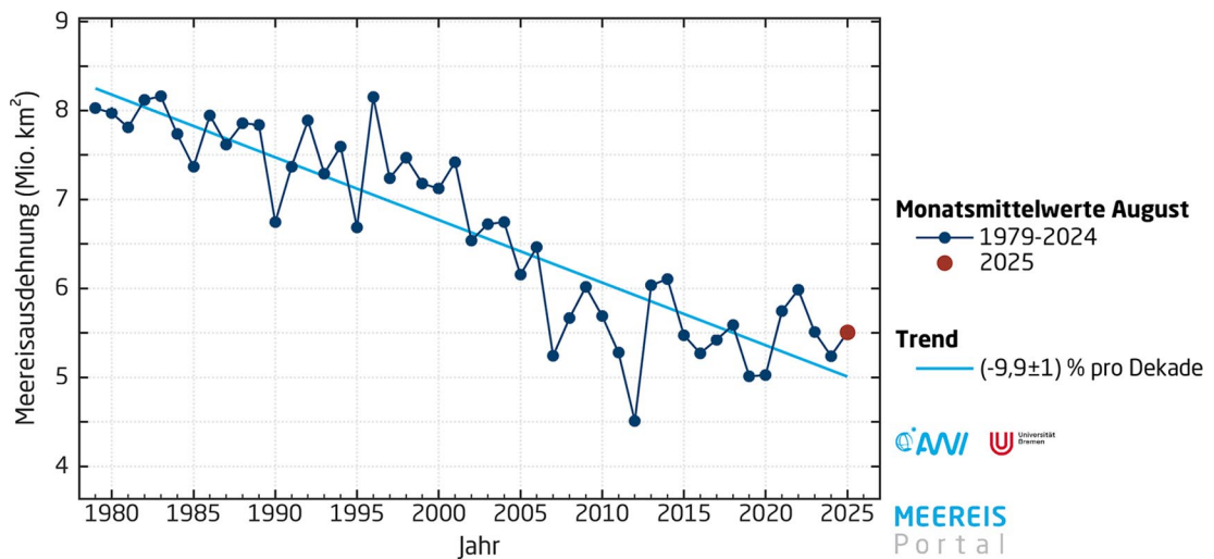
Abbildung 3: Mittlere Meereisausdehnung in der Arktis
